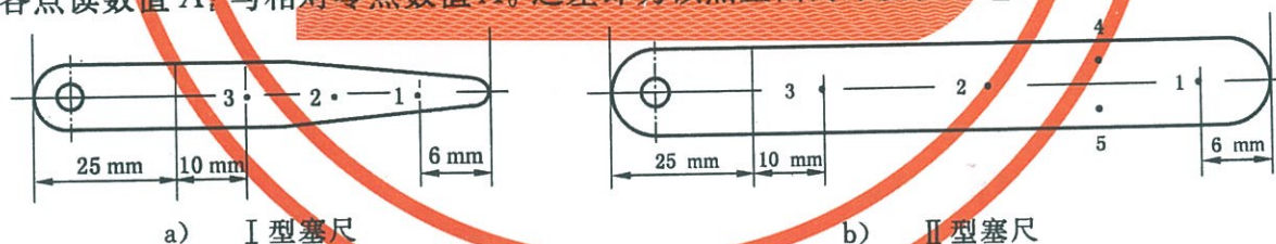
图 4 塞尺测量点示意图
