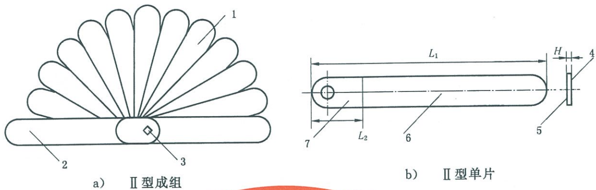
图2 II型塞尺结构示意图
