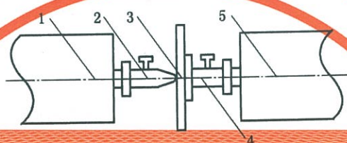
图 3 塞尺厚度测量示意图
