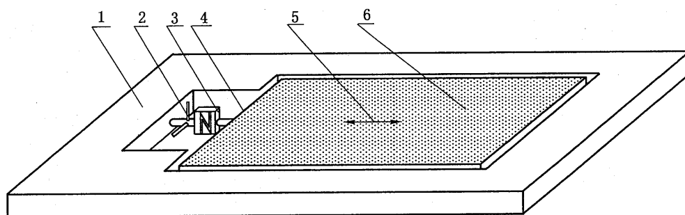
图 1 检定示意图
