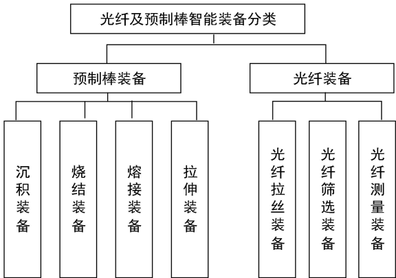
图1 光纤及预制棒智能装备分类
